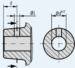
pinhole
